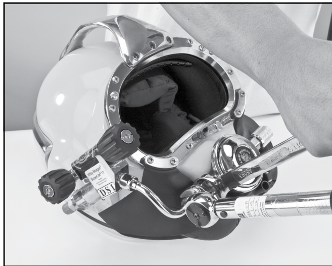
La contratuerca y el tubo curvado deben ajustarse según el par de apriete especificado.
