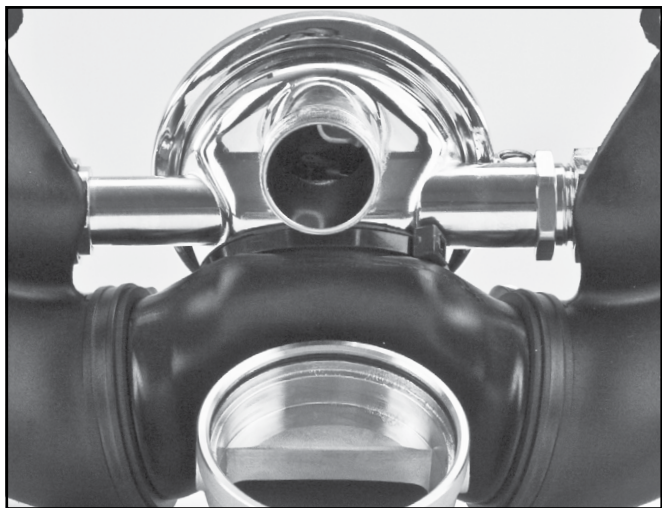
El sistema de escape Quad-Valve™ se debe conectar correctamente al regulador y a la cubierta con acople.
