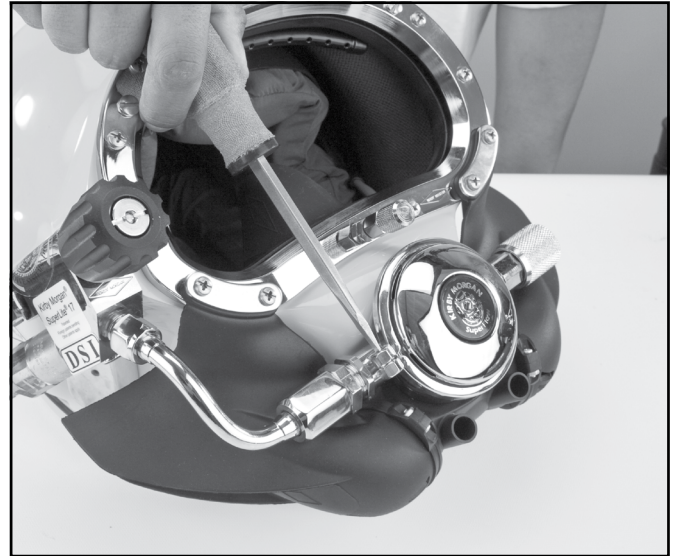
Retire la abrazadera del regulador a demanda.
