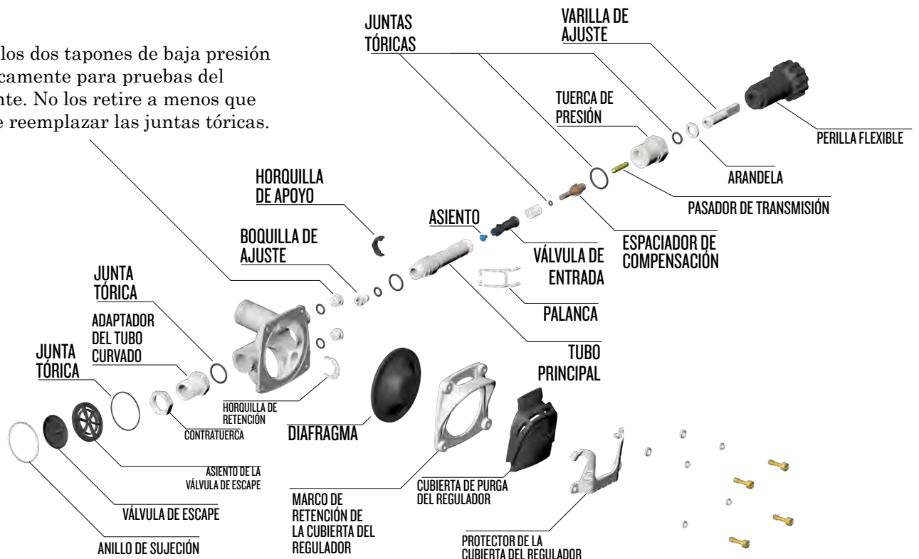
Vista despiezada del regulador compensado 455
