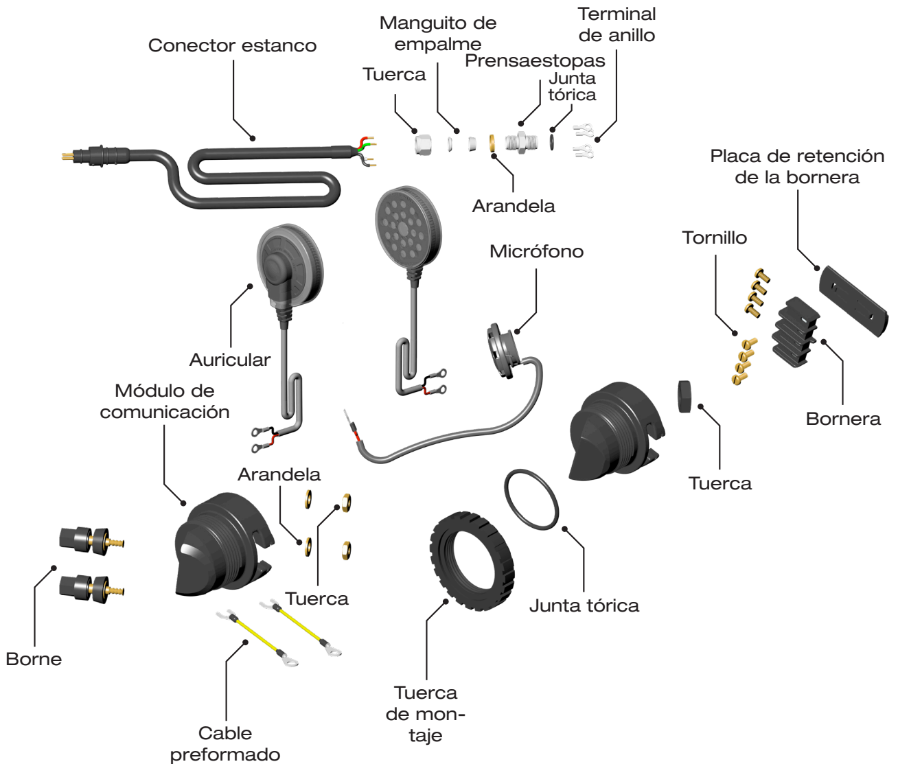
Componentes del sistema de comunicación (diseño nuevo)
