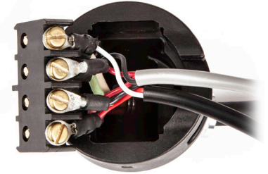
CONECTOR ESTANCO (MACHO) NUEVO
