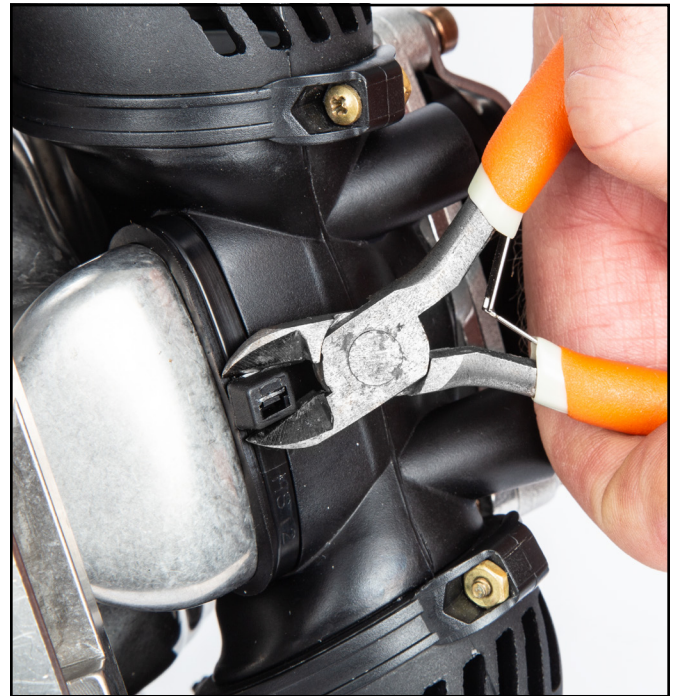
Corte el precinto que sujeta el cuerpo principal del sistema de escape Quad-Valve al tubo del conjunto de vaciado de agua en el casco.
