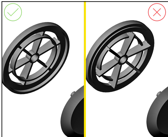
Instale la nueva válvula de escape (si es necesario) en el asiento. Asegúrese de colocar la válvula del lado correcto del asiento del escape.
