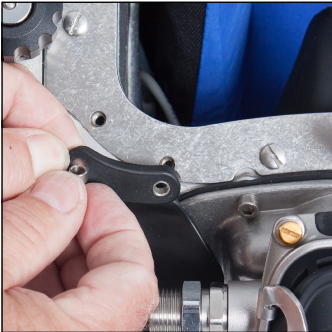
Asegúrese de retirar y dejar a un lado los espaciadores de las bigoterías.
