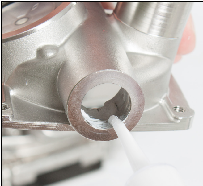
Aplique lubricante Christo-Lube® o similar al interior del regulador.
