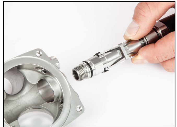
Presione los brazos de la palanca hacia abajo e instale cuidadosamente el conjunto del tubo principal en el cuerpo del regulador.
