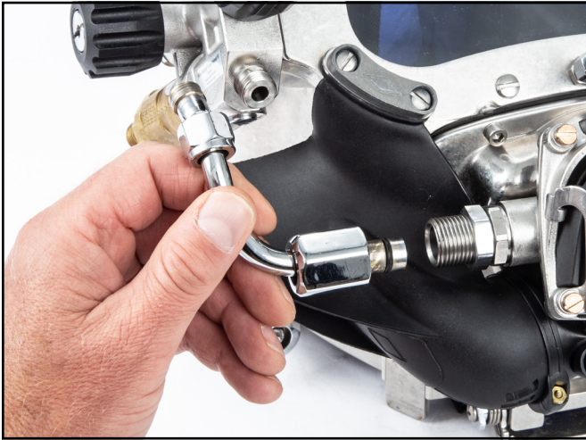
Retire el conjunto del tubo curvado.
