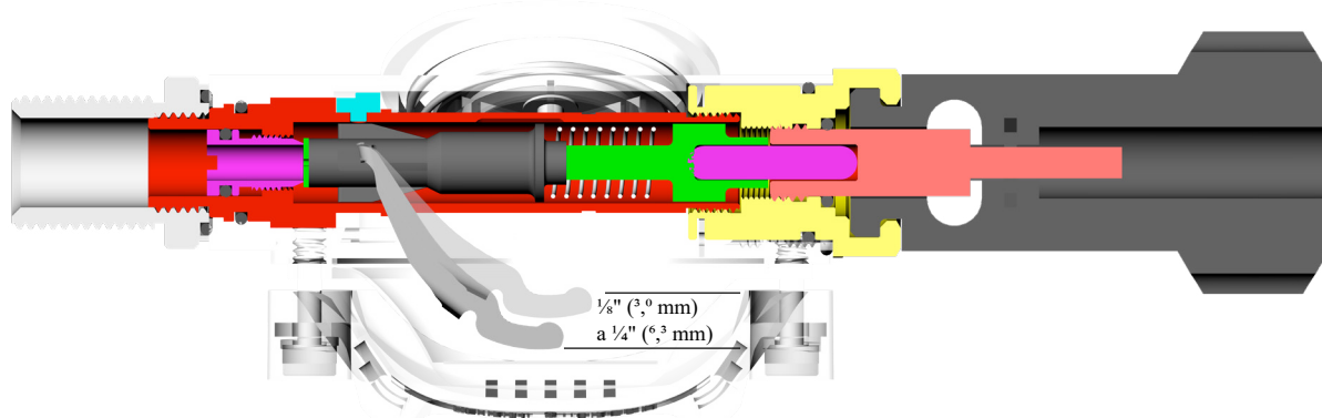
Diagrama del espacio libre máximo de los brazos de la palanca
