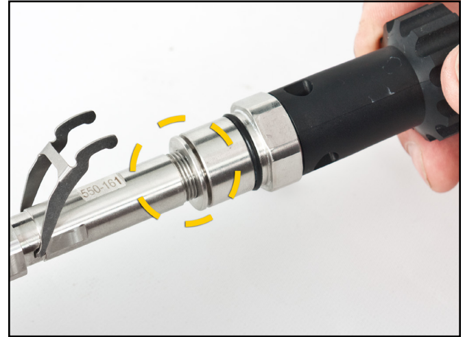
Al instalar el tubo principal en el cuerpo del regulador, es muy importante que queden expuestas más de tres roscas en el tubo principal.
