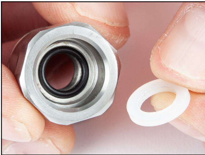
Coloque la junta tórica en el interior de la tuerca de presión de ajuste, seguida de la arandela de apoyo de la varilla.
