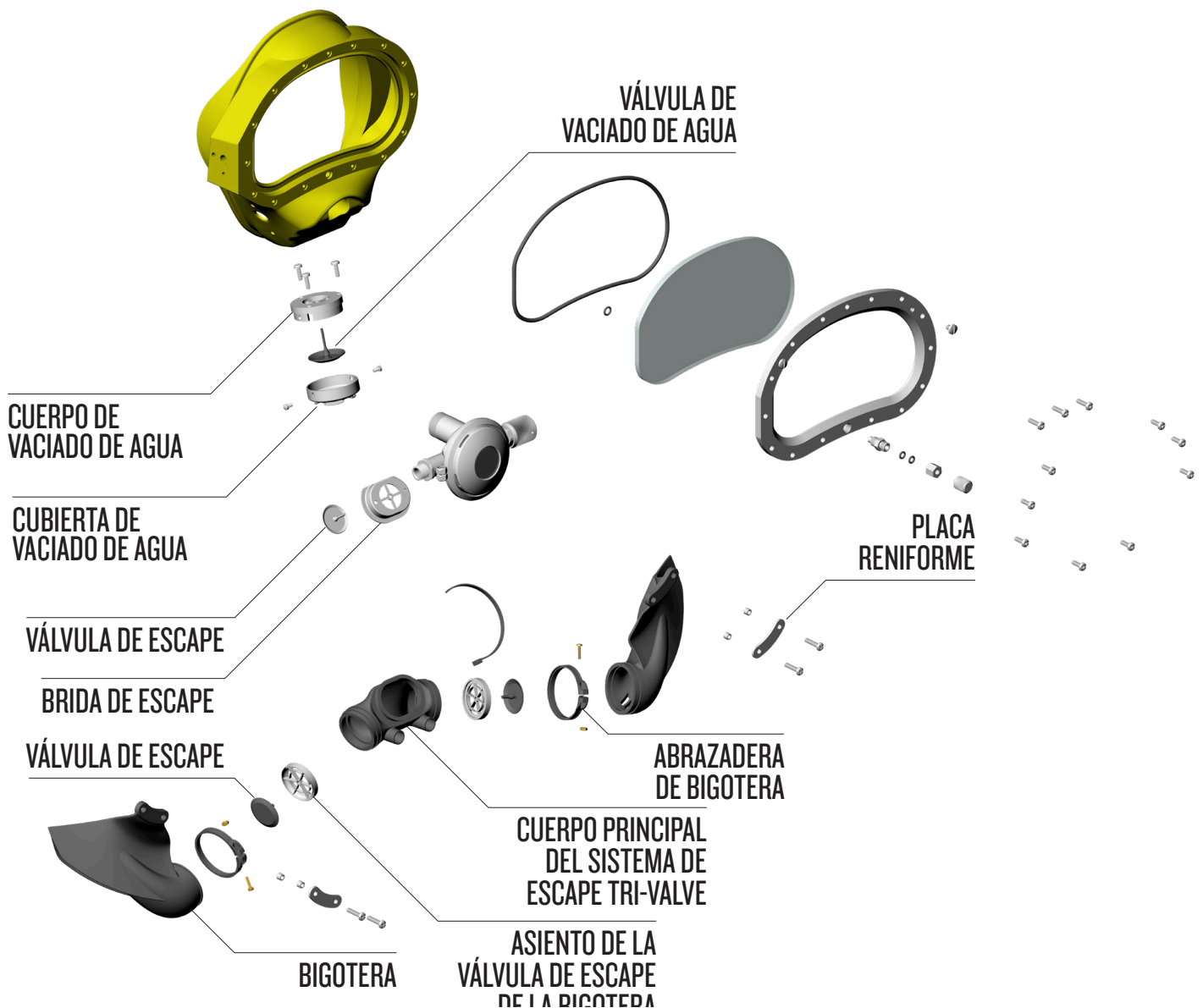
Vista despiezada del sistema de escape Tri-Valve de las máscaras BandMask
